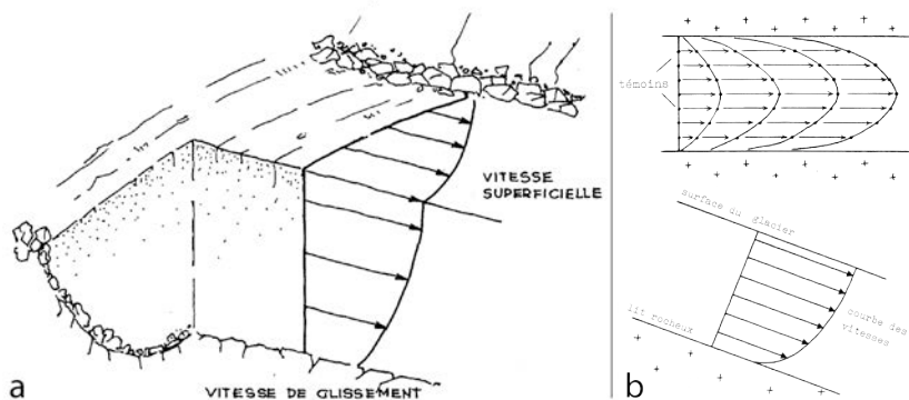
Fig. 5.12 : Répartition des vitesses de déplacement d'un glacier : a) schéma en perspective (Zryd, 2001) synthétisant b) deux schémas en plan et en coupe (Dorthe-Monachon, 1987).
